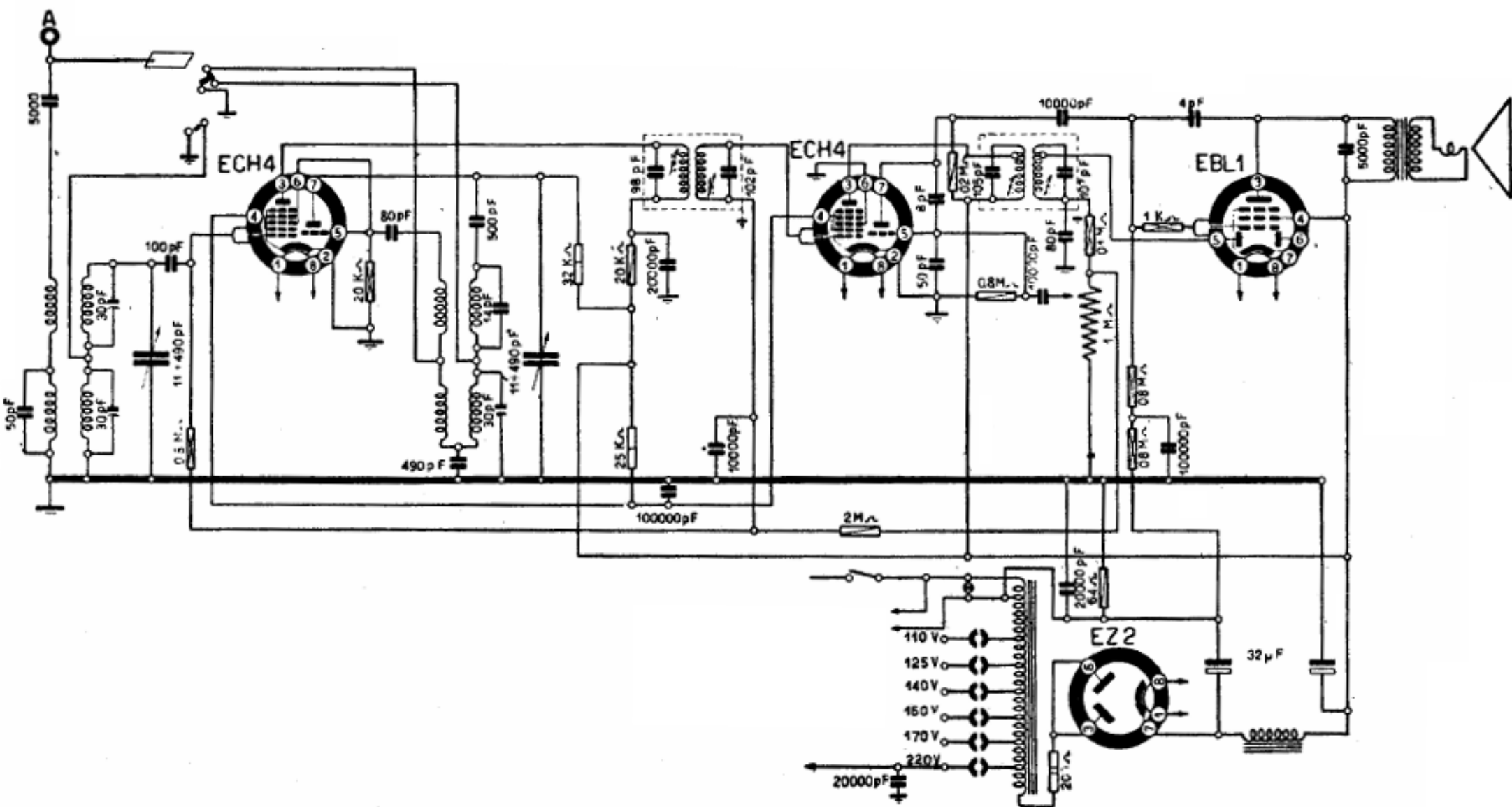
PHILIPS - Mod. BI 270 A - Piccola supereterodina con due ECH4 simile ai modelli BI 460/A e HI 470/A. Media frequenza: 468 kc/s. Per taratura v. norme modelli indicati. Produzione 1946-47.
